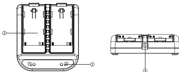
①充电指示灯 ②电池充电通道 ③DC输入接口
